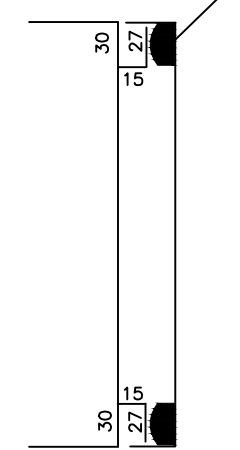
BURLETE DE GOMA DE 25 mm
