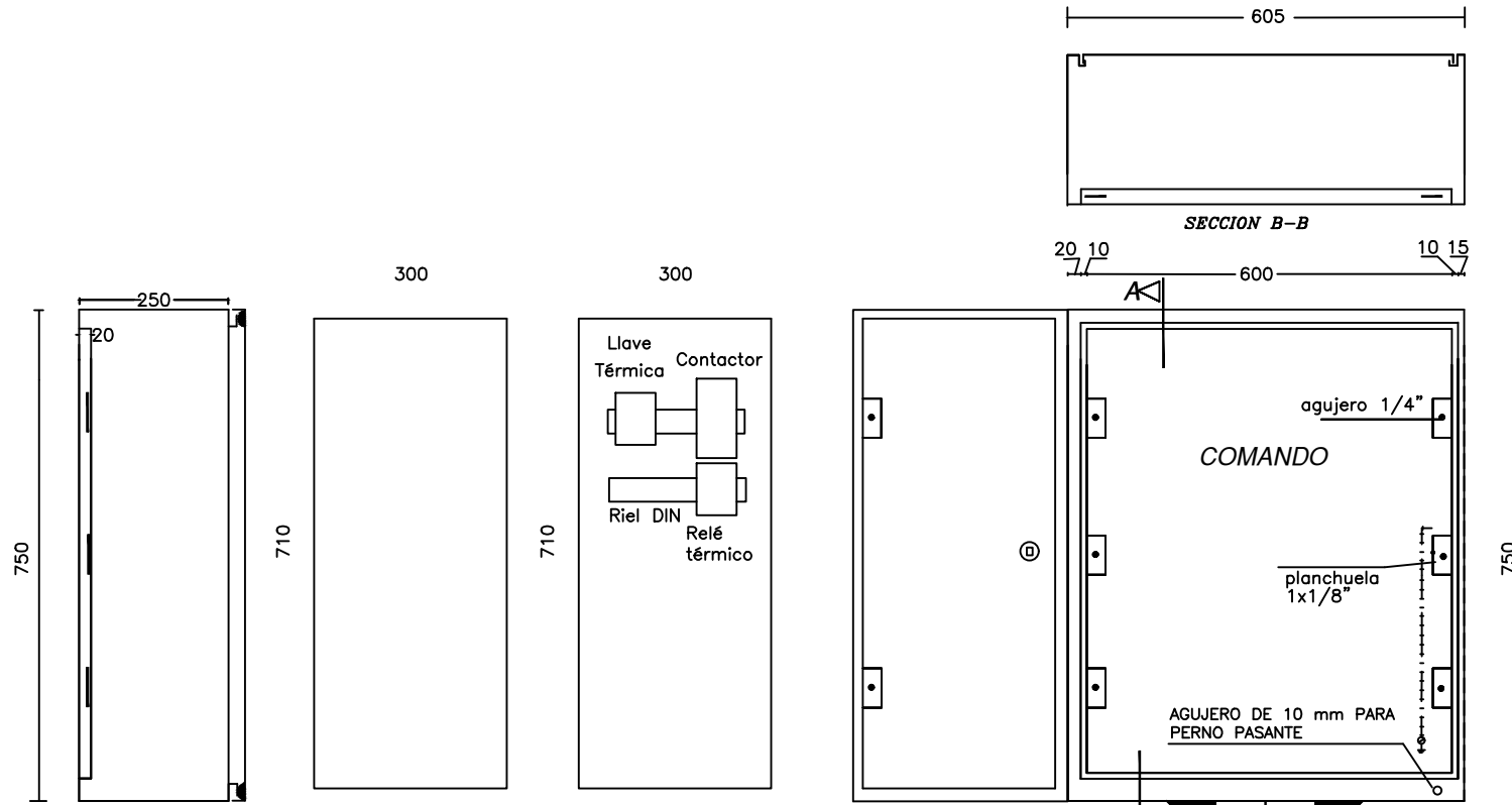
Bandeja para elementos de protección y comando
