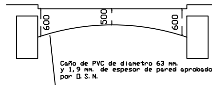
DETALLE ENTRE CAJAS
