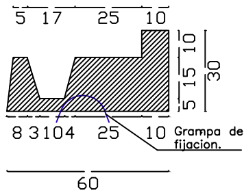
DETALLE A (marco)
