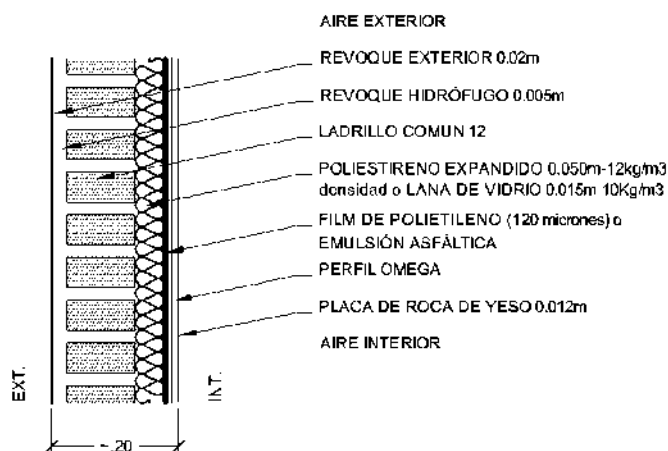
MURO DE LADRILLO COMÚN DE 12 + AISLACIÓN (6 CAPAS) K=0.57 W/m 2 K
