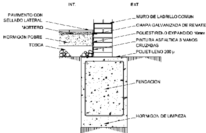
APOYO DE MURÓ SOBRE CIMENTACION
