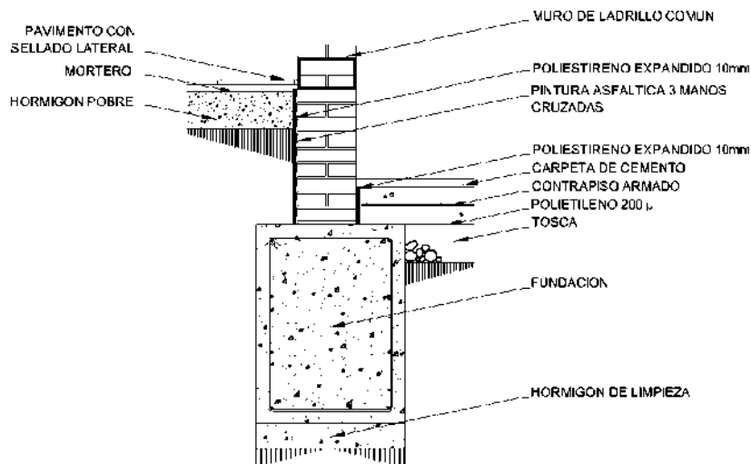
MURÓ DE SOTANO
