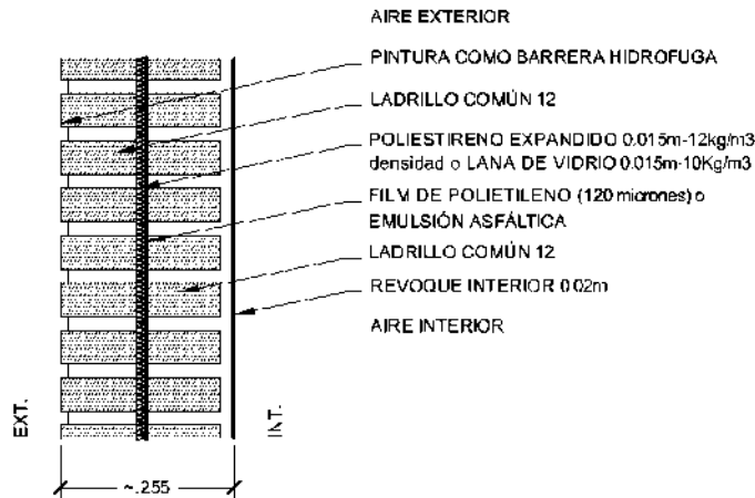
MURO DOBLE LADRILLO COMÚN DE 12 + AISLACIÓN (6 CAPAS) K=1.13 W/m 2 K
