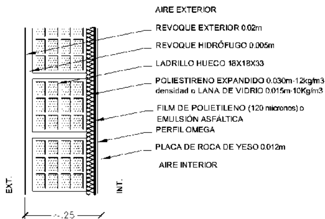
MURO DE LADRILLO HUECO DE 18 + AISLACIÓN (6 CAPAS) K=0.60 W/m 2 K
